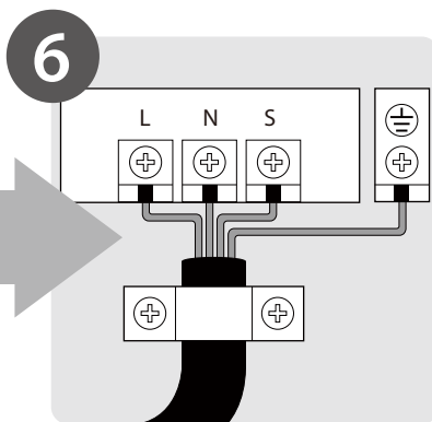
6 Podłączenie okablowania (Strona 17)
