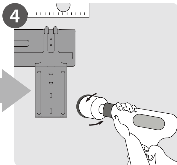
Wiercenie otworu w ścianie (Strona 12)
